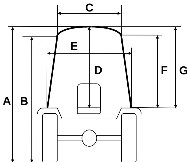
Cabina “COMPACT” NEW HOLLAND T3.80F Gommatura posteriore Trattore 360/70 R.24
