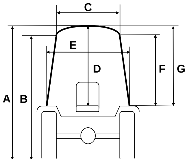
Cabina “COMPACT” NEW HOLLAND T4.100F S Gommatura posteriore Trattore 380/70 R.24
